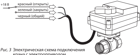
Рис. 3 Электрическая схема подключения крана с электроприводом серии Neptun Bugatti Pro 18 B
