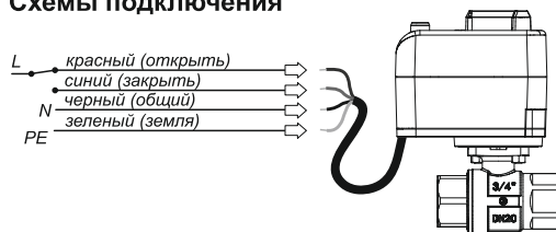
Электрическая схема подключения крана с электроприводом серии Neptun Profi Click 230B (рис. 3)
