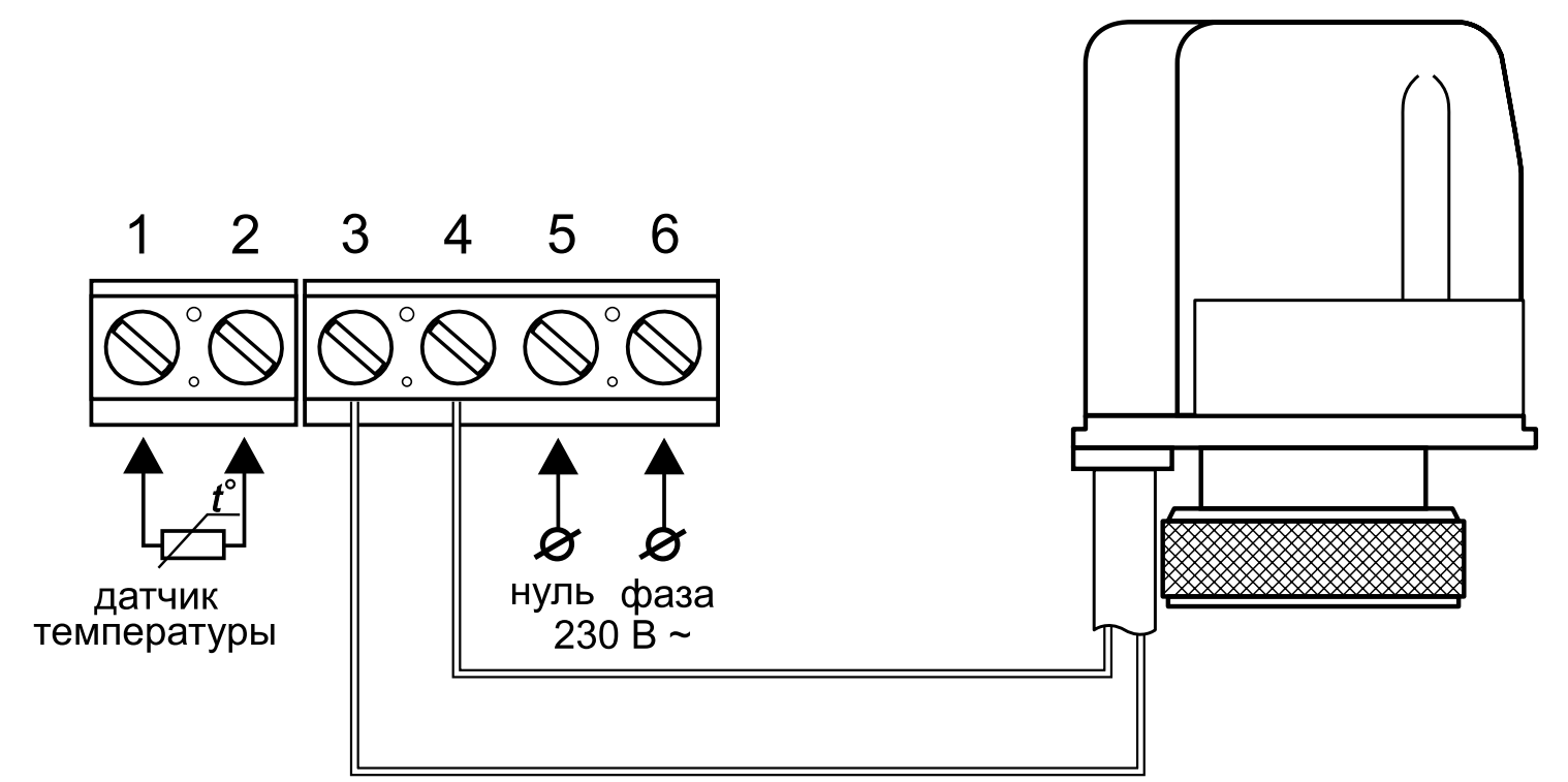
Рис. 3 Схема подключения термостатической ГОЛОВКИ
