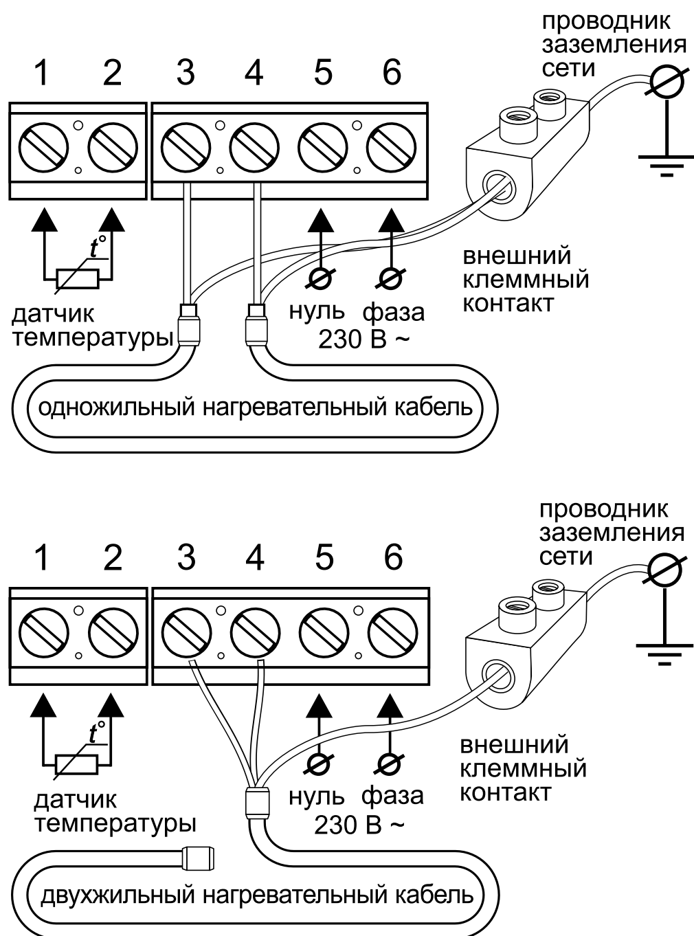
Рис. 2 Клеммный контакт терморегулятора
