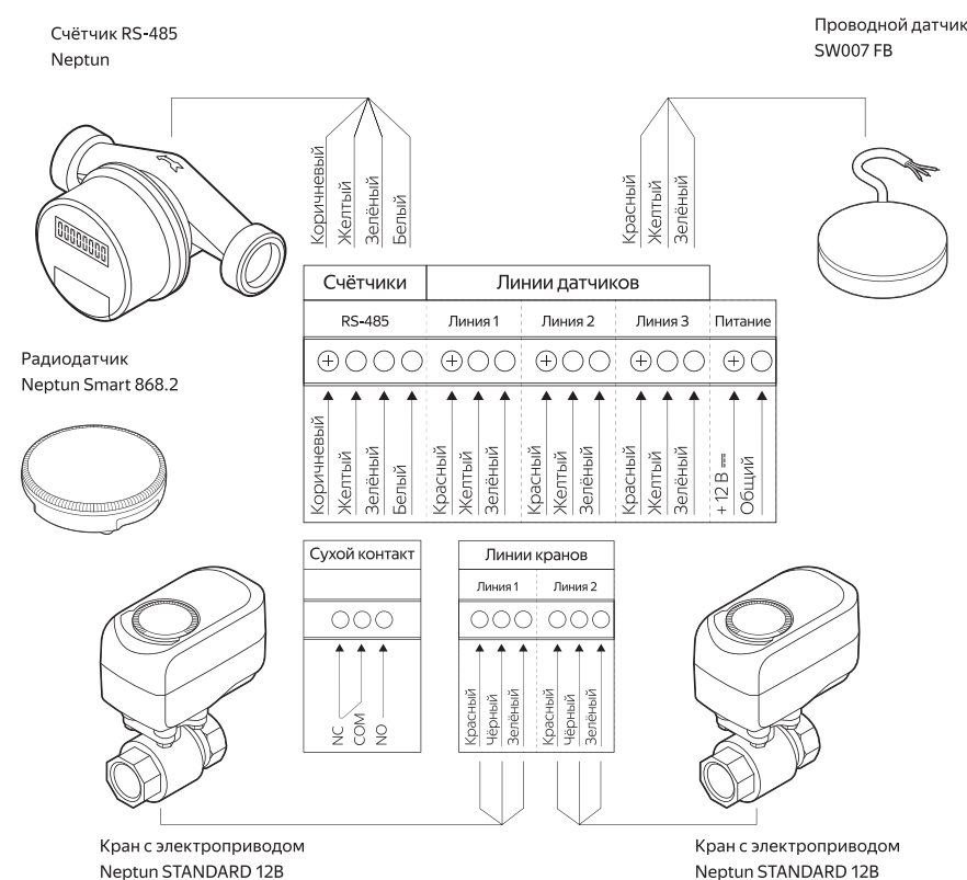
Рисунок 6. Схема подключения
