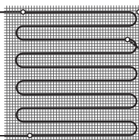
1-сүр. Маттын конструкциясы
