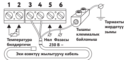
2-сүр. Матты электр тармагына туташтыруу схемасы
