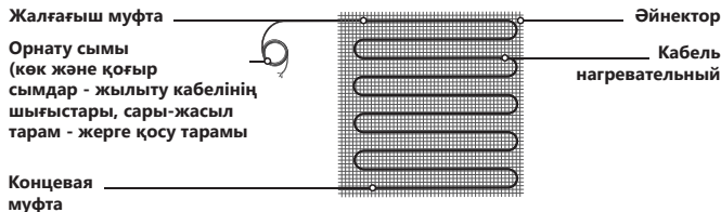
1-сур. Төсеніш конструкциясы
