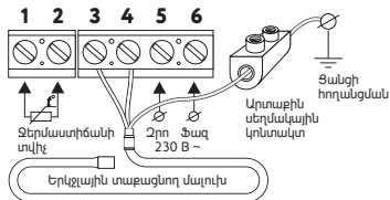
Նկ 2. Էլեկտրական ցանցին ներքևակի միացման սխեմա
