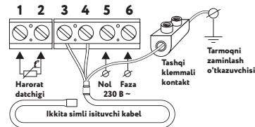
2-rasm. To'shakni elektr tarmog'iga ulash sxemasi
