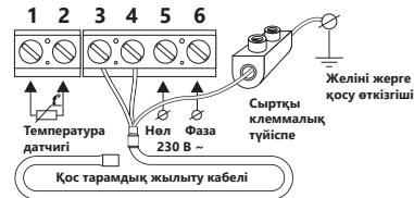
2-сур. Төсенішті электр желісіне қосу схемасы
