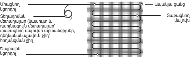
Նկ 1. Ներքնակի կառուցվածքը
