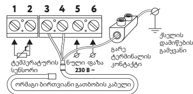
სურ. 2. ელექტრო ქსელში ხალიჩის შეერთების სქემა
