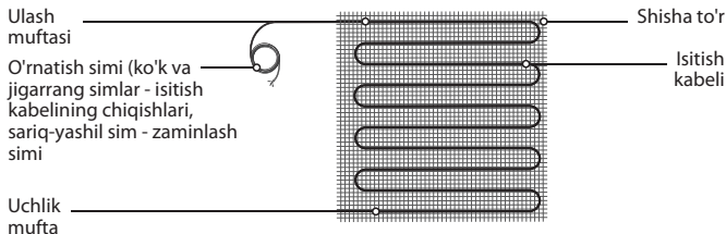
1-rasm To'shakning tuzilishi
