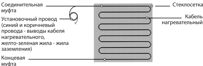
Рис. 1. Конструкция мата
