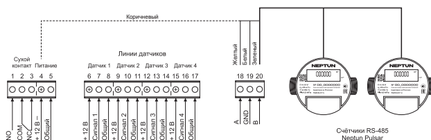
Рис. 2. Подключение счетчиков к модулю управления
