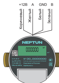
Рис. 1. Назначение проводов
