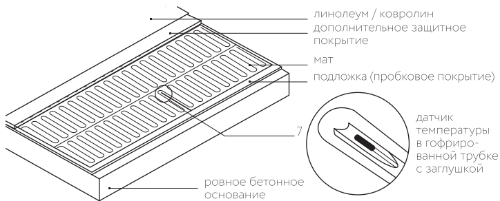
Рисунок 7. Конструкция элементов пола с использованием в качестве финального покрытия линолеума или ковролина
